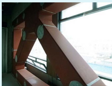
3Q-Brace工法
