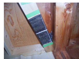
②炭素繊維シート巻き補強
