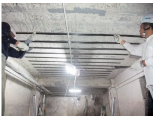
スラブ補強例
