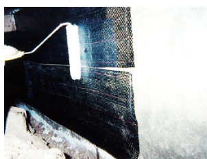
①炭素繊維シート貼付け
