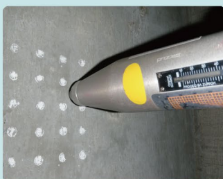
シュミットハンマー （コンクリート強度試験）
