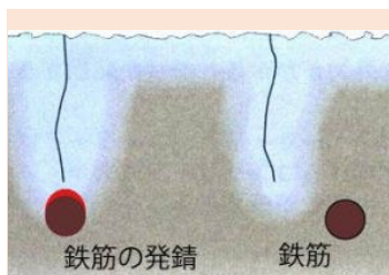
低圧エポキシ樹脂注入工法
