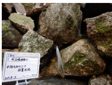
⑦水抜き加工シート設置完了
