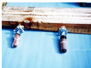
①エポキシ樹脂試験注入
