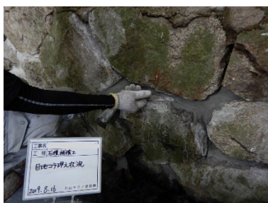
⑪目地コテ押さえ
