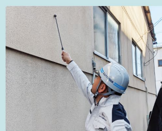
パルハンマー （浮き部打診点検）
