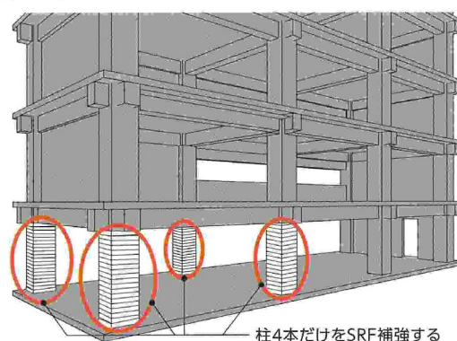
耐震実験例（東大地震研究所と共同実験）
